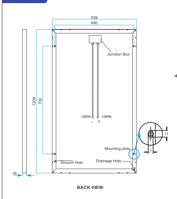
MCA-100
